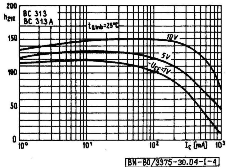
Rys. I-4. Zależność statycznego współczynnika wzmocnienia prądowego od prądu kolektora h_{21E} = f(I_c)
