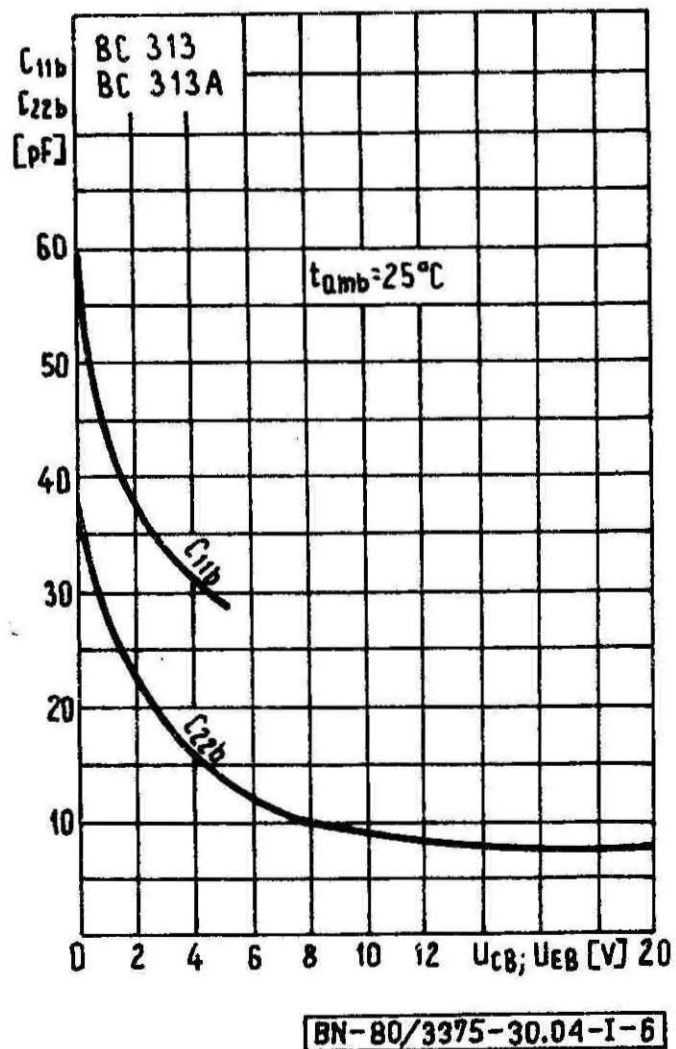
Rys. I-6. Zależność pojemności złączy od napięcia C_{EBO} = f(U_{EBO}) , C_{CBO} = f(U_{CBO})
