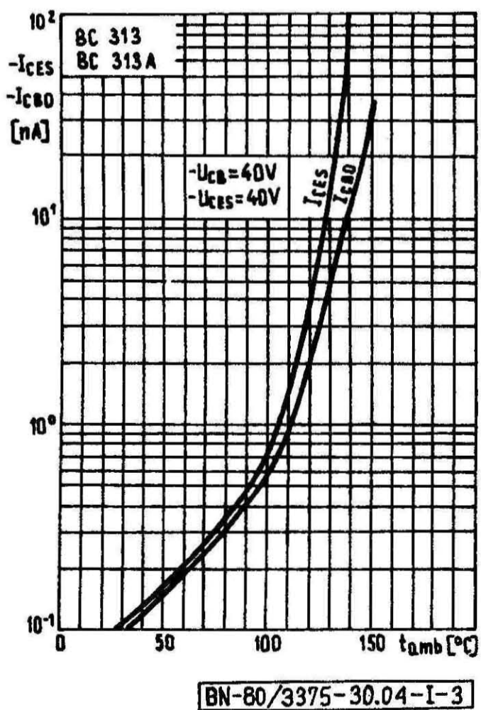
Rys. I-3. Zależność temperaturowa prądów zerowych I_{cES} I_{cBO} = f(t_{amb})
