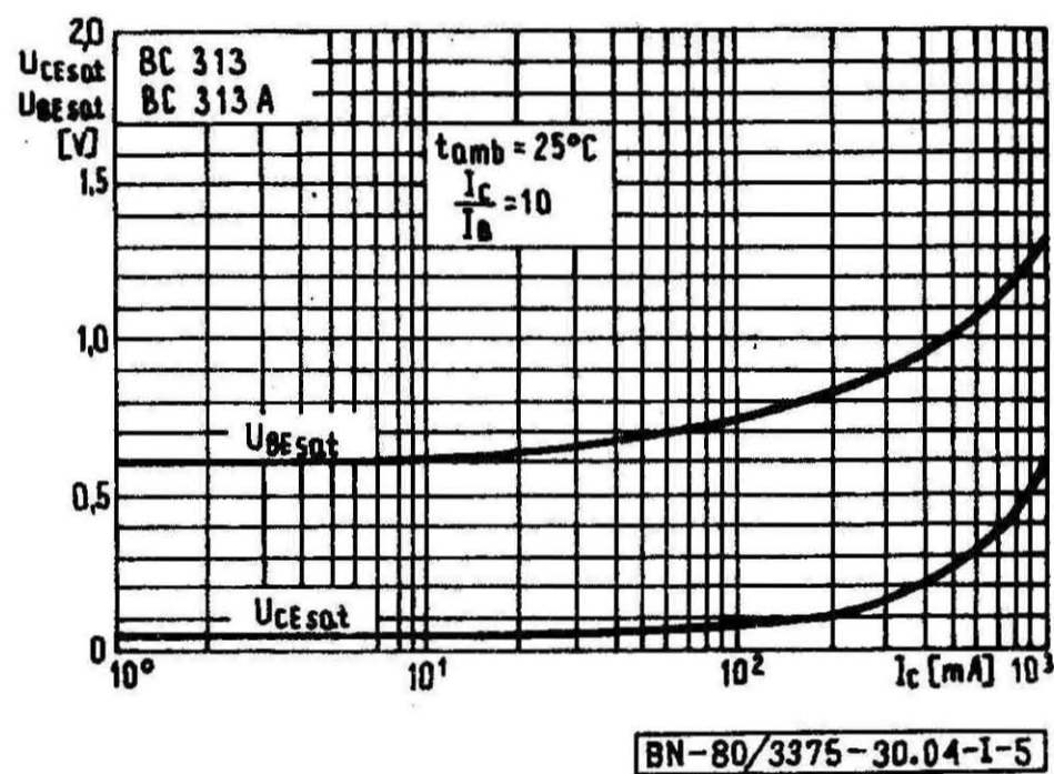
Rys. I-5. Zależność napięcia nasycenia od prądu kolektora U_{ce sat} = f(I_c)
