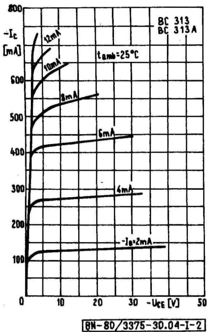
Rys. I-2. Charakterystyka wyjściowa I_c = f(U_{ce}) I_b — parametr
