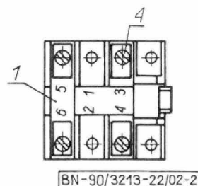
Rys. 2. Numeracja zacisków
