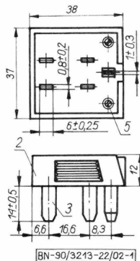
Rys. 1. Przykładowa konstrukcja wtyczki WT-4
