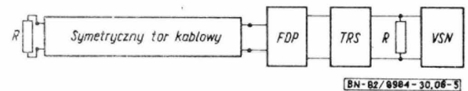
Rys. 5. Pomiar szerokopasmowy wartości skutecznej napięcia zakłóceń: FDP — filtr dolnoprzepustowy taki sam jak w układzie pomiarowym na rys. 4, TRS — transformator symetryzujący w paśmie częstotliwości od 300 \text{ Hz} do częstotliwości granicznej FDP lub wyższej, o impedancji falowej wejścia i wyjścia 600 \Omega , VSN — miliwoltomierz wartości skutecznej przebiegów niesinusoidalnych o wejściu niesymetrycznym (pozostałe warunki jak dla VSS na rys. 4), R — rezystor 600 \Omega
