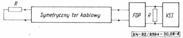
Rys. 4. Układ do pomiaru wartości skutecznej napięcia zakłóceń: VSS — miliwoltomierz wartości skutecznej przebiegów niesinusoidalnych o wejściu symetrycznym, FDP — filtr dolnoprzepustowy, R — rezystor 600 \Omega
