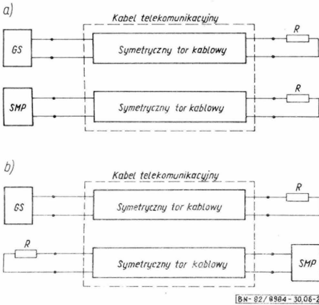
Rys. 2. Układ do pomiaru tłumienności przenikowej a) przenik zbliżony, b) przenik zdalnego: GS — generator sygnałów sinusoidalnych o impedancji wewnętrznej 600 \Omega , SMP — selektywny miernik poziomy, R — rezystor 600 \Omega
