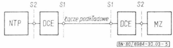
Rys. 5. Układ do pomiaru zniekształceń telegraficznych NTP — nadajnik tekstu pomiarowego (CCITT, V52), DCE — urządzenie komunikacyjne transmisji danych, MZ — miernik zniekształceń telegraficznych
