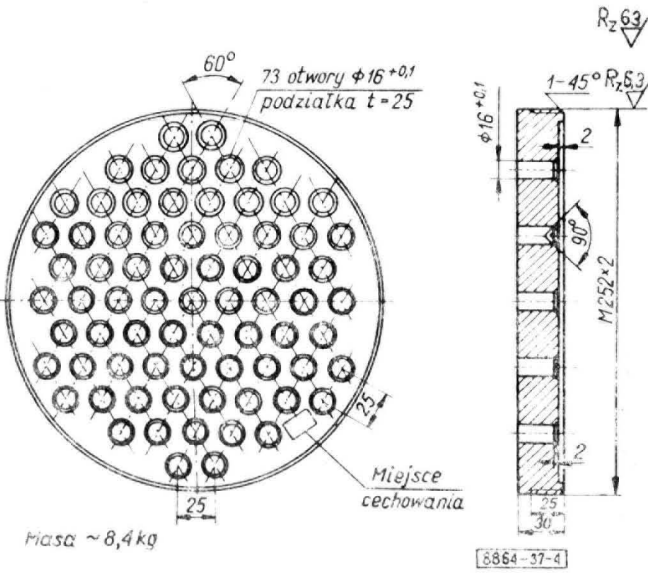
Rys. 4. Płyta sitowa węzownicy wymiennika WCO
