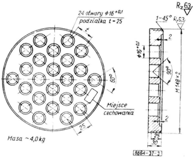
Rys. 3. Płyta sitowa węzownicy wymiennika WCO
