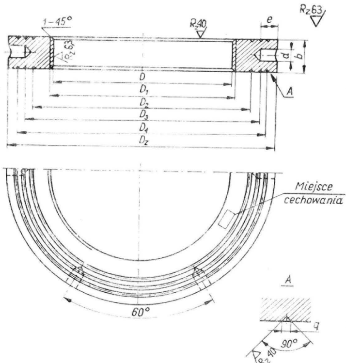
Rys. 7. Nakrętka wymiennika WCO
