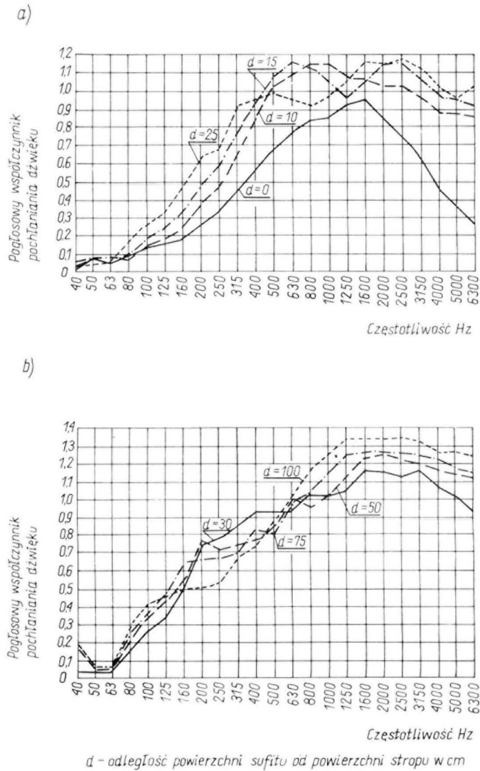
Rys. 12. Charakterystyki pogłosowego współczynnika pochłaniania dźwięku sufitu kasetonowego (komora otwarta)
