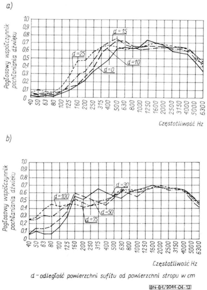
Rys. 13. Charakterystyka pogłosowego współczynnika pochłaniania dźwięku sufitu kasetonowego (komora zamknięta)
