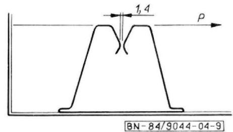
Rys. 9. Schemat działania siły rozchylającej
