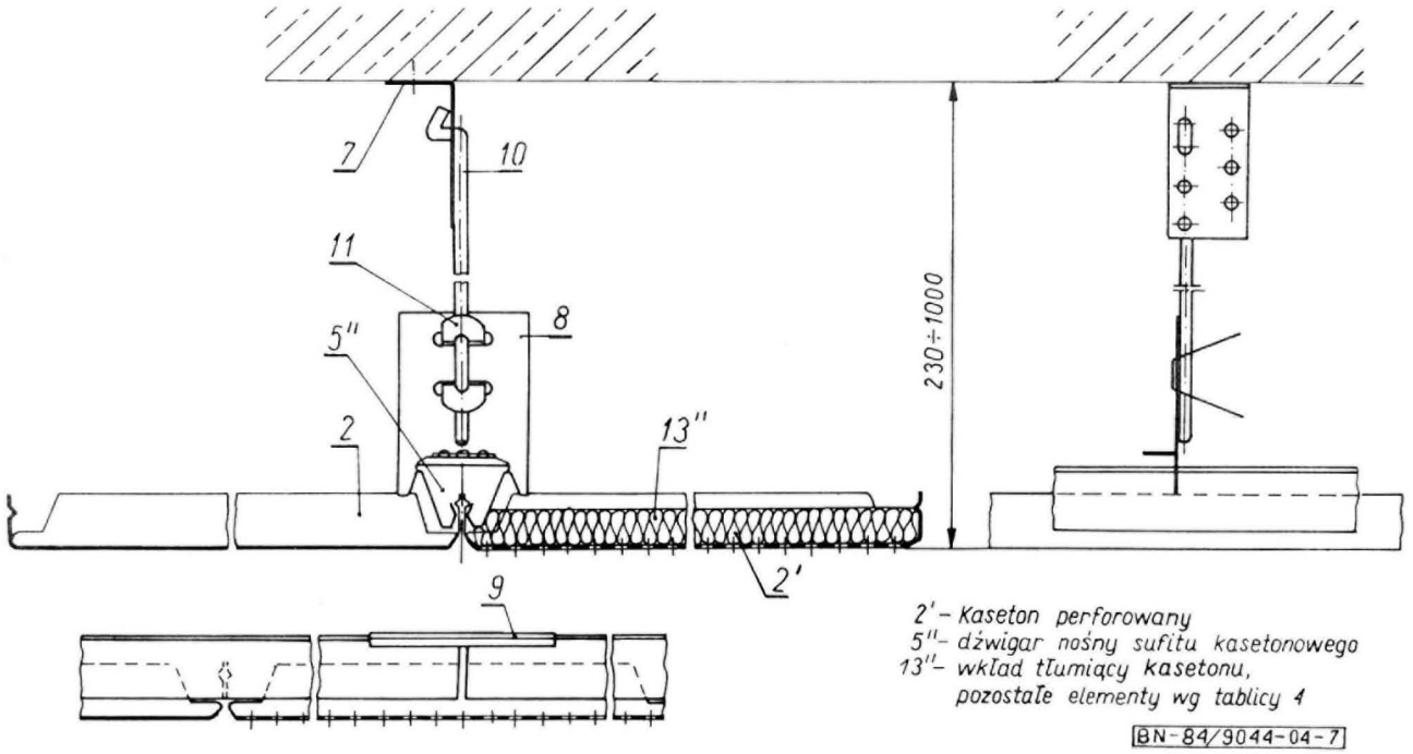
Rys. 7. Sufit podwieszany kasetonowy
