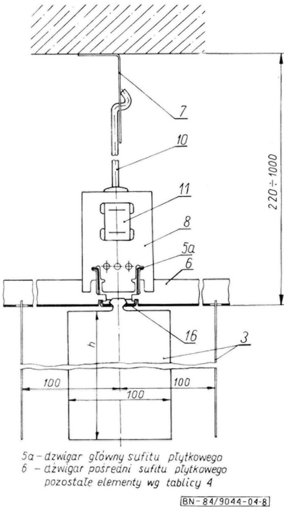
Rys. 8. Sufit podwieszany płytkowy
