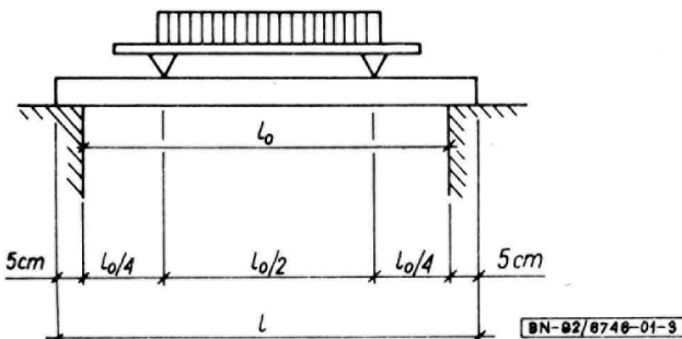
Rys. 3. Schemat obciążenia płyt przy badaniu nośności
