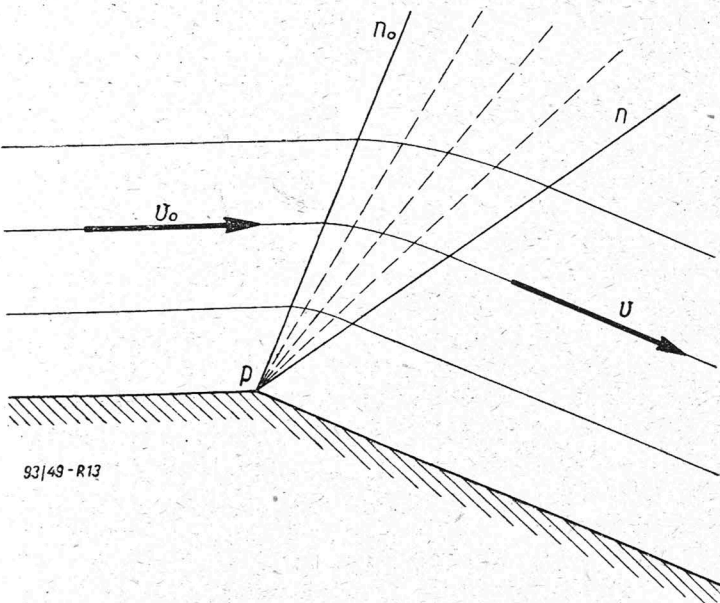
Rys. 13. Linie prądu oraz wachlarz rozrzedzeń przy opływie załamania wypukłego.
