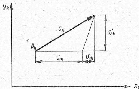
Rys. 10. Odwzorowanie podobne Prandtla.
