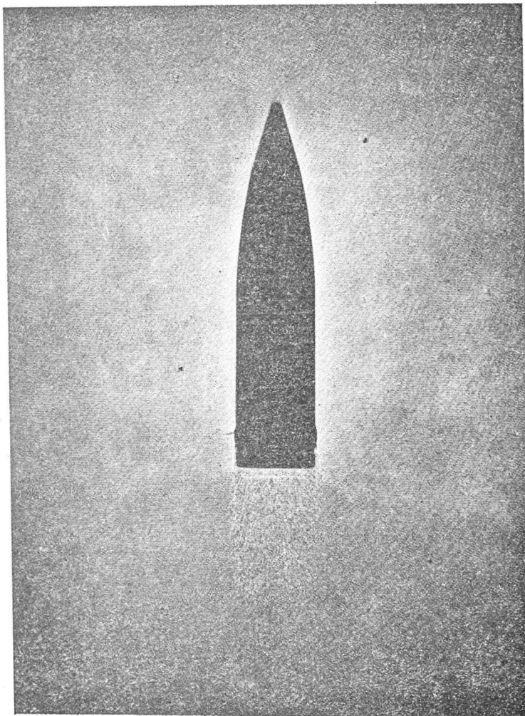
Rys. 1. Przepływ poddźwiękowy przy M = 0,86 . Widoczny tylko obszar zaburzeń poza pociskiem.
