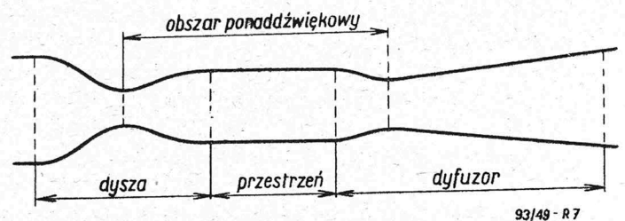
Rys. 7. Ukształtowanie przewodu przemian.
