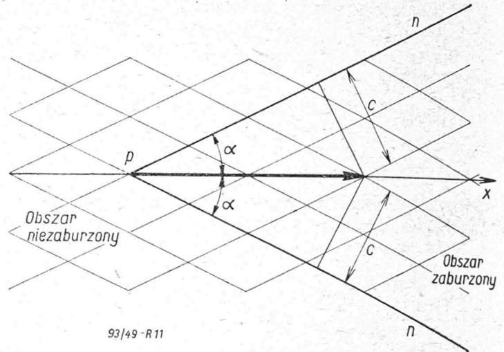
Rys. 11. Siatka Macha.
