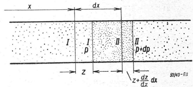
Rys. 8. Zmiany ciśnienia pod wpływem impulsu.
