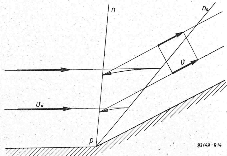
Rys. 14. Pozbawione fizycznego sensu teoretyczne linie prądu przy opływie załamania wklęsłego.
