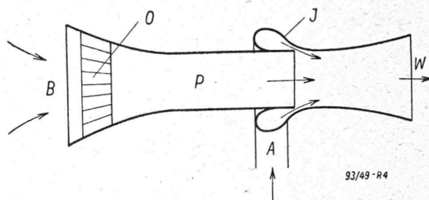
Rys. 4. Schemat tunelu o napędzie pośrednim.
