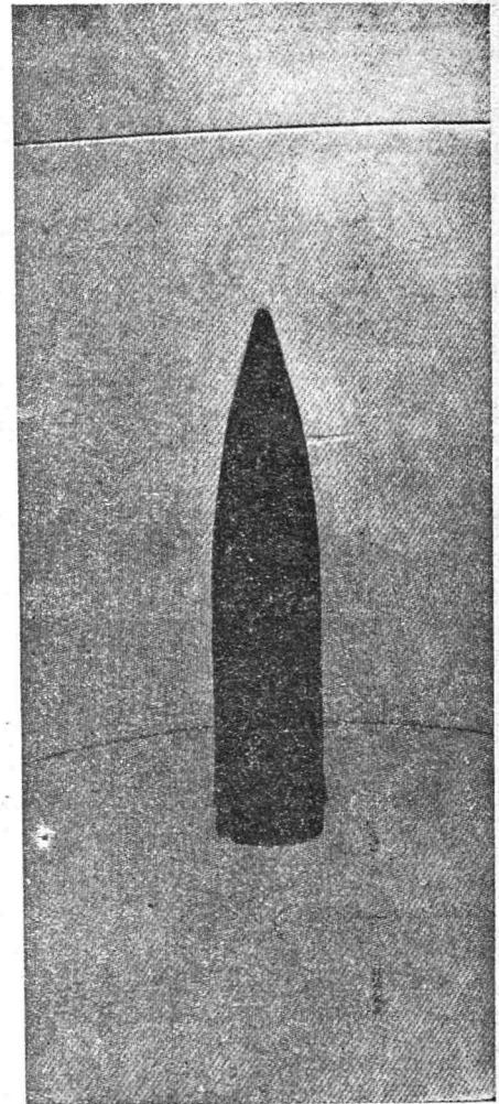
Rys. 2. Przepływ z prędkością dźwięku M = 1,01 . Przed pociskiem pojawia się „fala czołowa” w postaci linii nieciągłości ciśnienia. Na boku pocisku tworzy się miejscowa linia zgęszczenia 1) .
