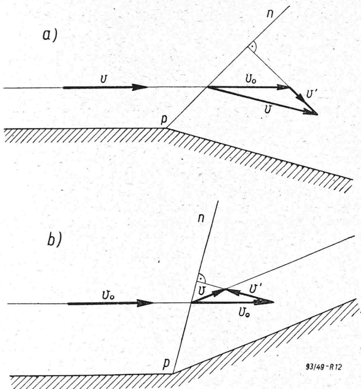
Rys. 12. Przepływ na załamaniach: a) wypukłym, b) wklęsłym.
