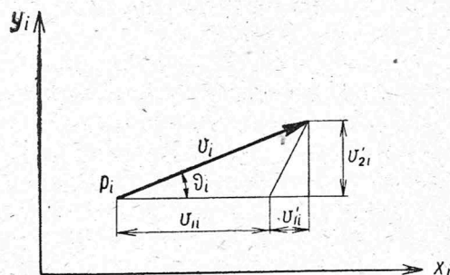
Rys. 10. Odwzorowanie podobne Prandtla.
