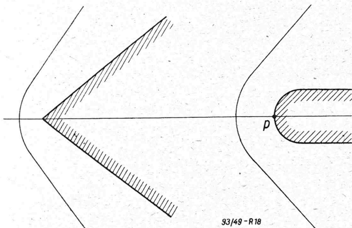
Rys. 18. Kształt linii zgęszczenia przed tępej klinem i przed tępej przeszkodą.
