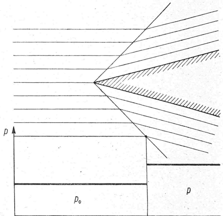
Rys. 16. Opływ ponaddźwiękowy klina i rozkład ciśnień wzdłuż linii prądu.
