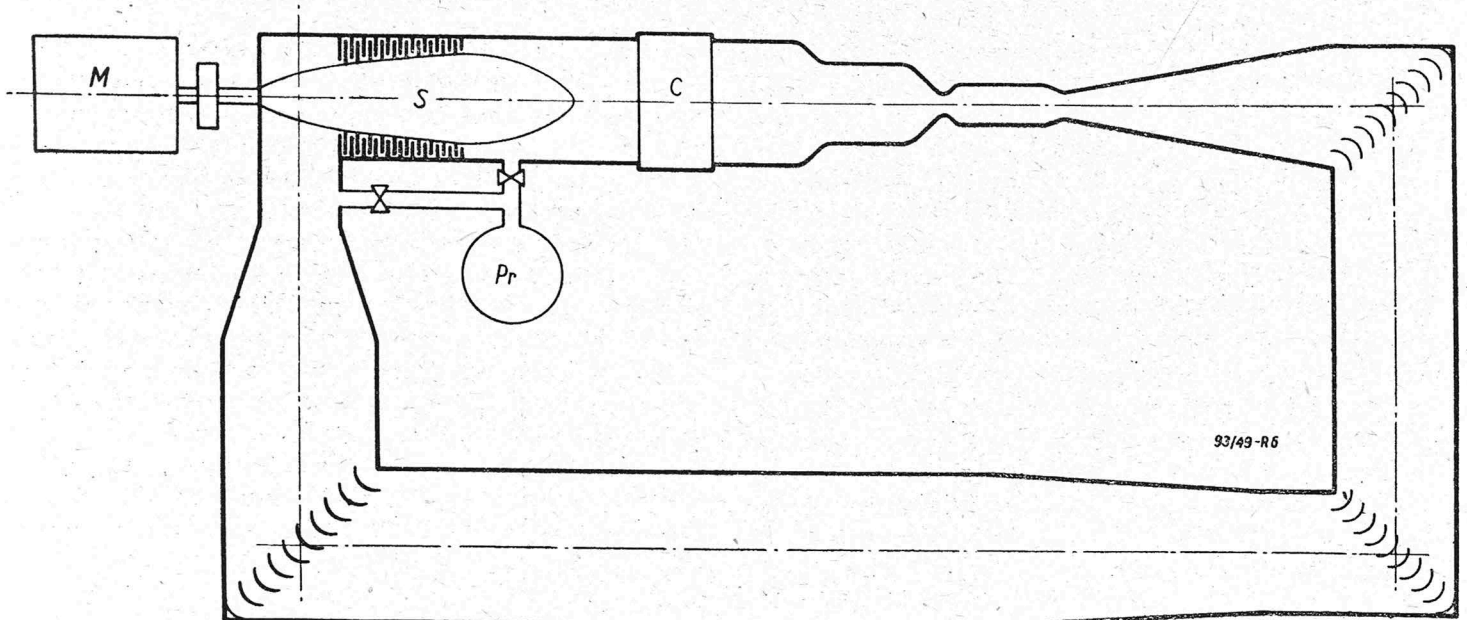
Rys. 6. Schemat tunelu o działaniu ciągłym.
