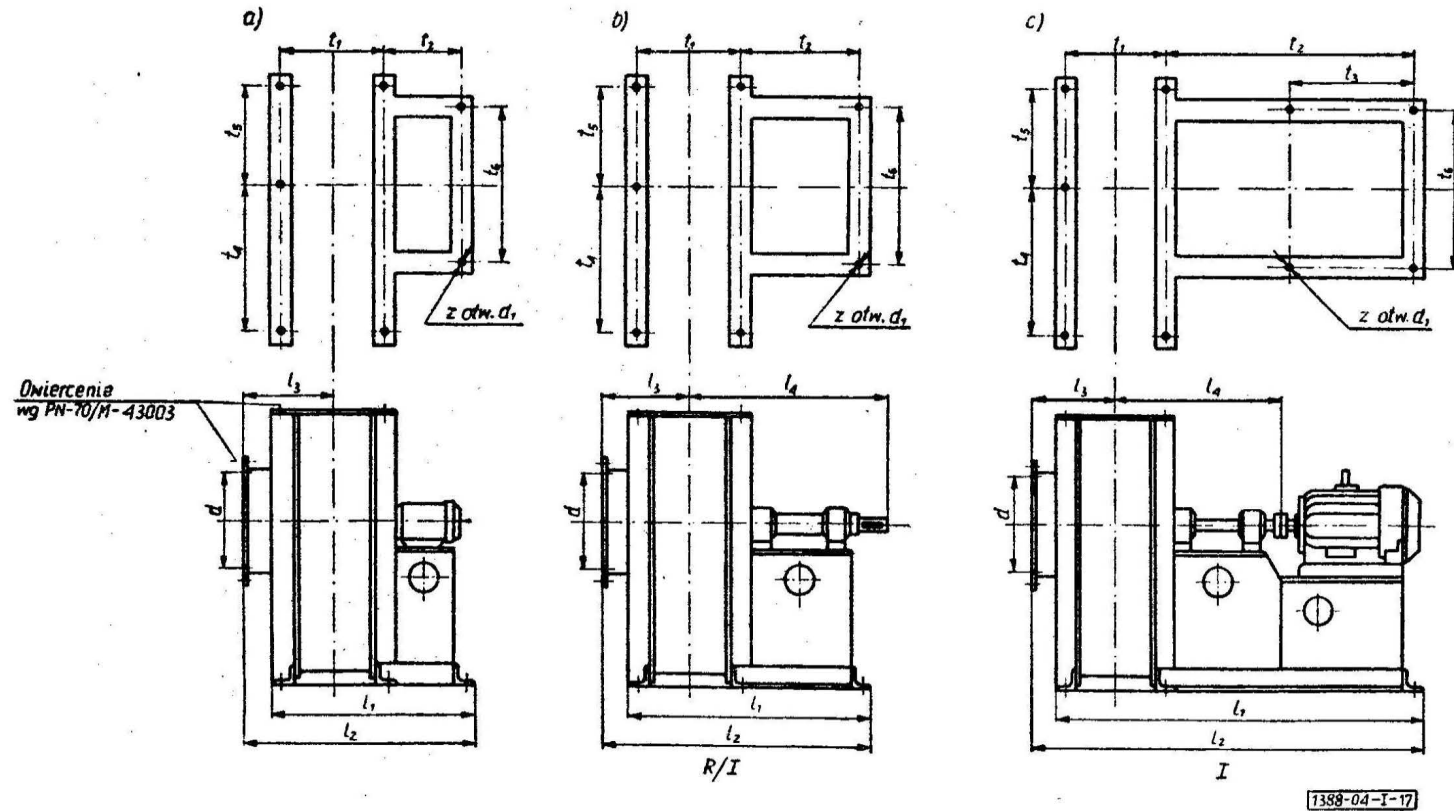
Rys. I-17. Główne wymiary wentylatorów promieniowych
