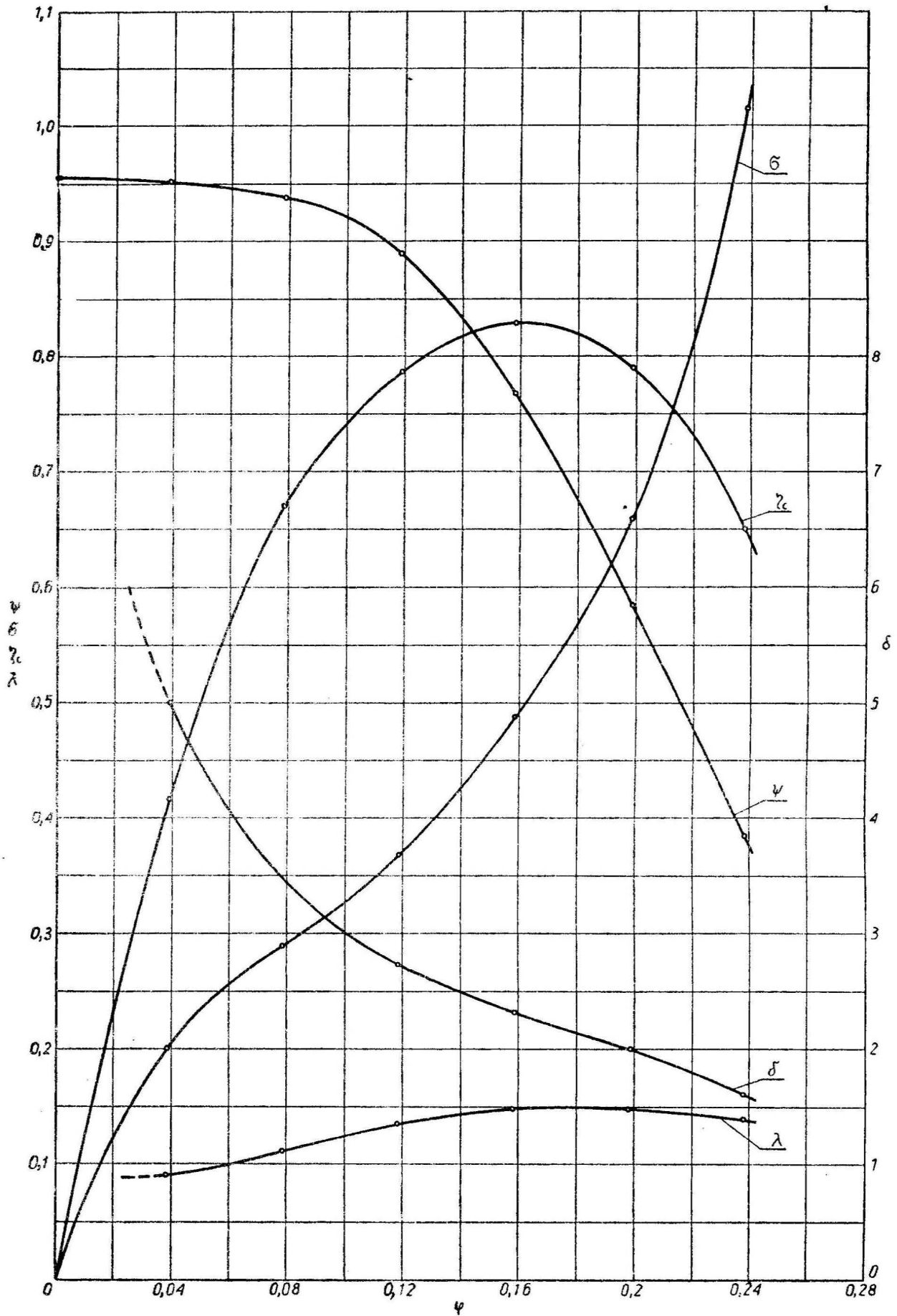
Rys. I-7. Charakterystyka aerodynamiczna bezwymiarowa wentylatora bez regulacji
