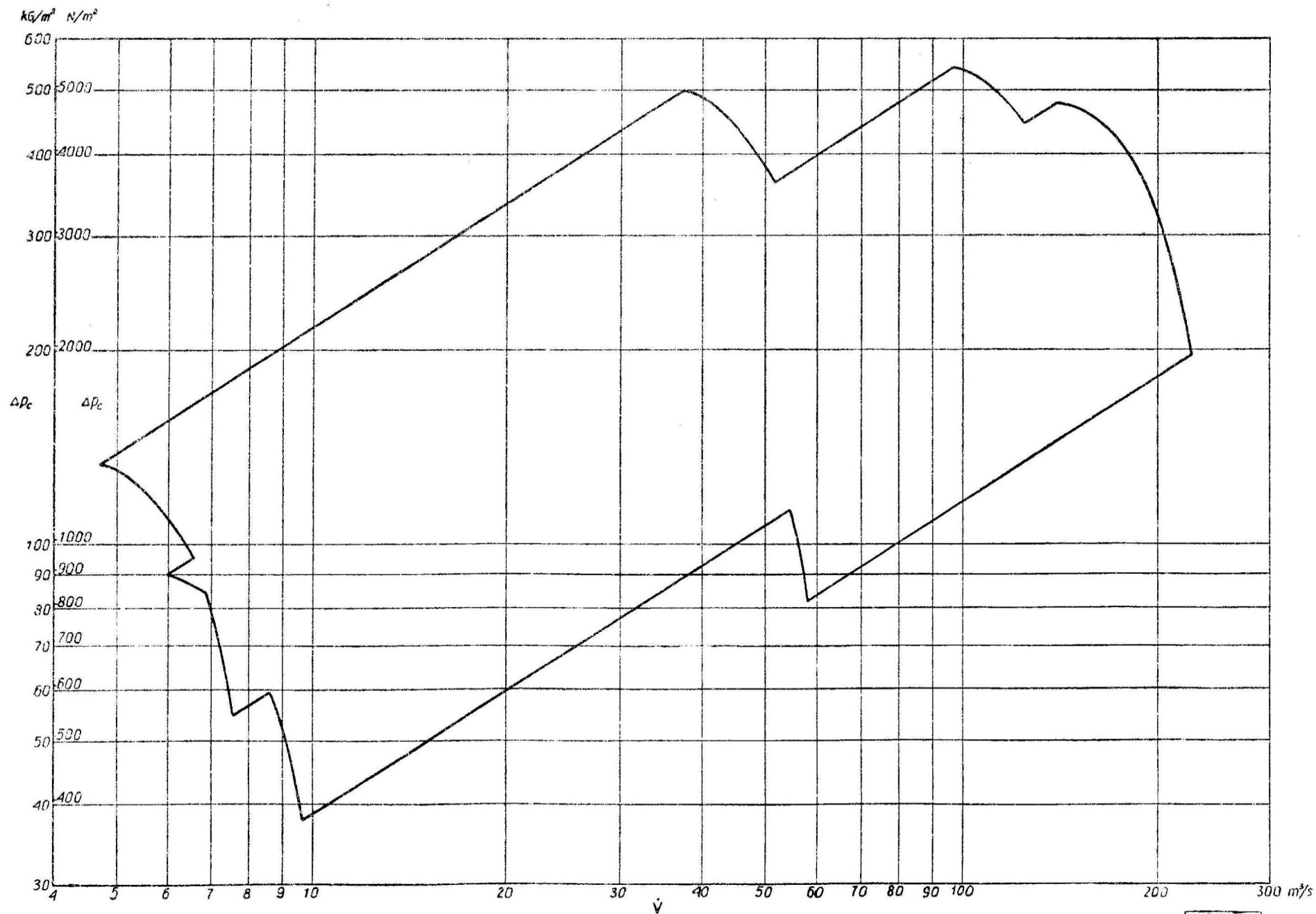
Rys. I-5. Uproszczona charakterystyka zbiorcza typoszeregu wentylatorów
