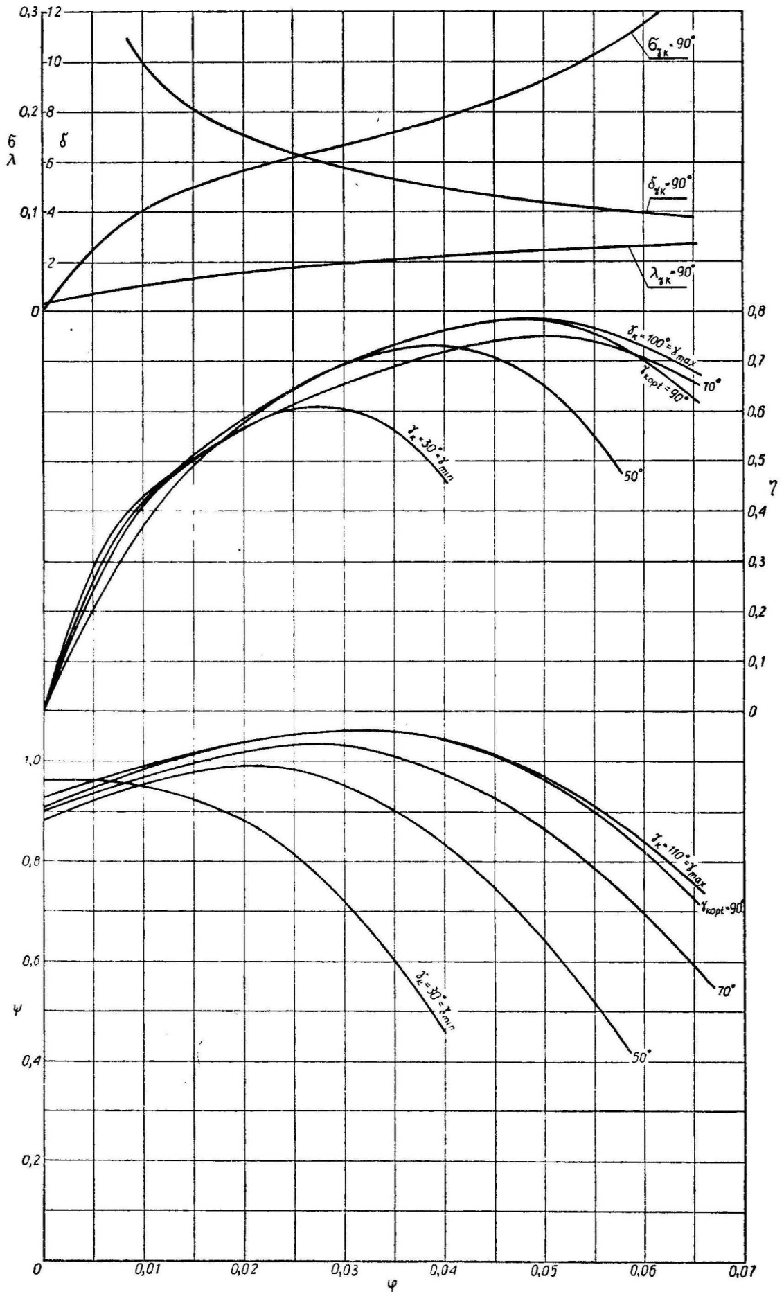
Rys. I-8. Charakterystyka aerodynamiczna bezwymiarowa wentylatora z regulacją za pomocą zmiany kąta ustawienia łopatek kierownicy przedwirlkowej
