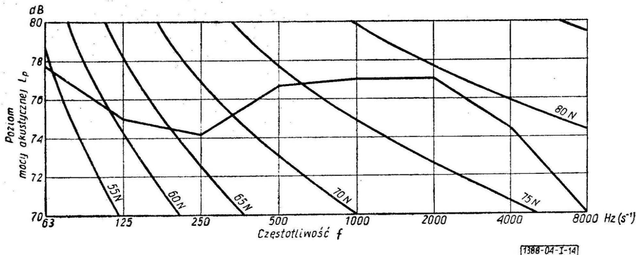
Rys. I-14. Widmo poziomu mocy akustycznej wentylatora przy optymalnej wydajności \dot{V} = 0,8, \text{ m}^3/\text{s} i prędkości obrotowej n = 2860 \text{ obr/min}
