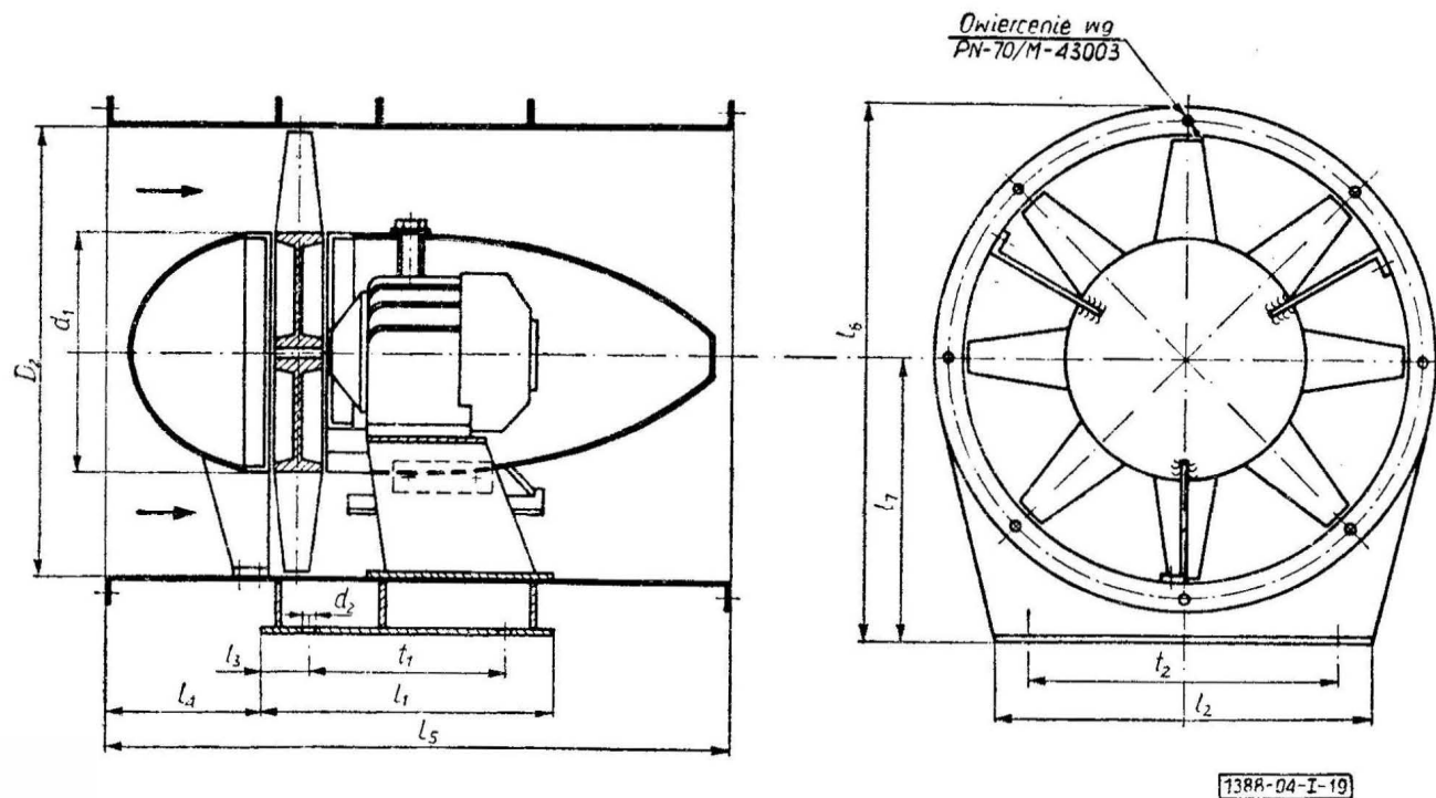
Rys. I-19. Główne wymiary wentylatorów osiowych
