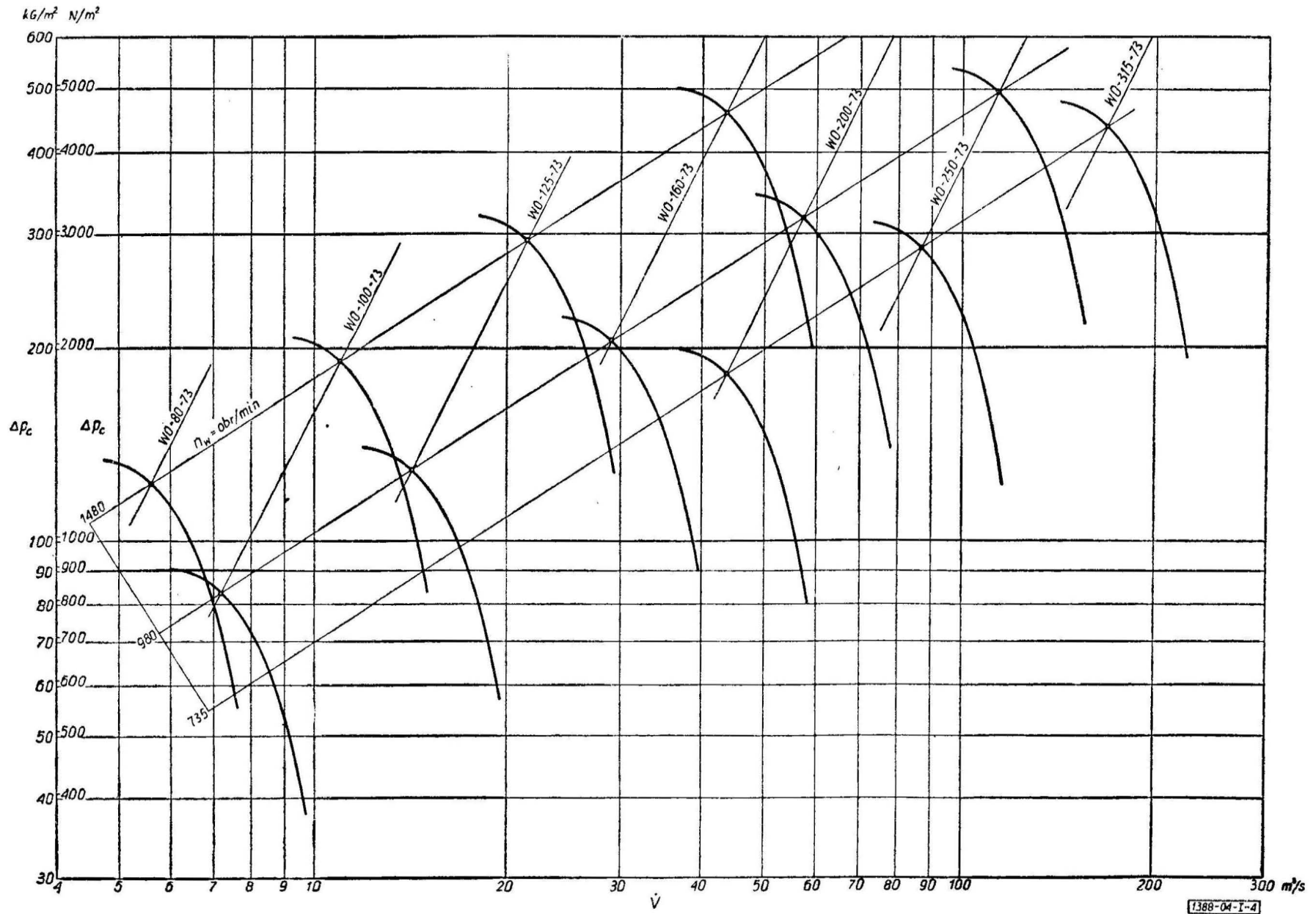
Rys. I-4. Aerodynamiczna charakterystyka zbiorcza typoszeregu wentylatorów
