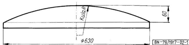
Rys. 1. Dennice do łączenia spawaniem (S)
