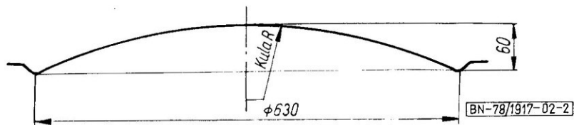
Rys. 2. Dennice do łączenia zakładkowego (Z)
