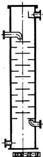
Rys. 18. Kolumna z przegrodami współśrodkowymi
