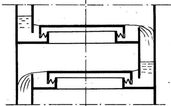
Rys. 3. Kolumna półkowa
