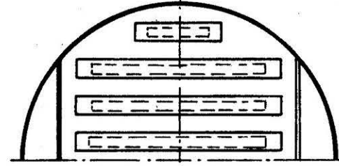
Rys. 5. Półki z tunelami o przekroju prostokątnym
