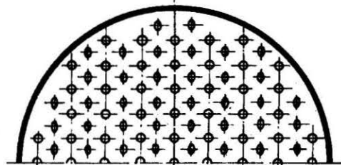
Rys. 10. Półki sitowe faliste 2230-02-10
