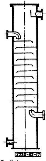
Rys. 17. Kolumna z przegrodami naprzemianległymi
