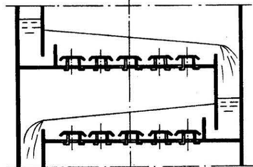
Rys. 5. Półki z tunelami o przekroju prostokątnym
