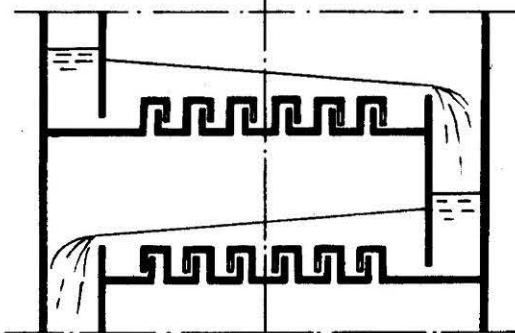
Rys. 4. Półki z kołpakami dzwonkowymi
