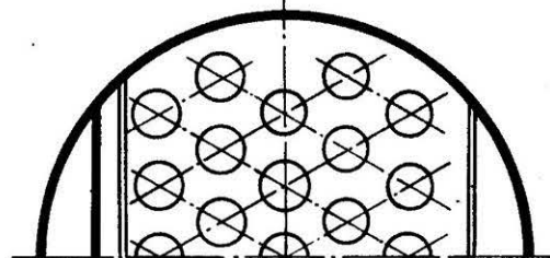
Rys. 7. Półki z zaworkami okrągłymi
