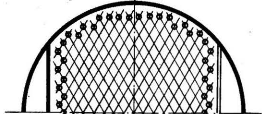
Rys. 9. Półki sitowe płaskie 2230-02-9
