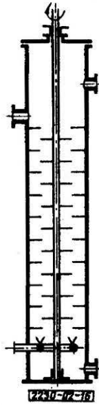
Rys. 16. Kolumna wirnikowa z wirującymi tarczami
