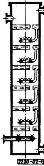
Rys. 19. Kolumna dyfuzorowa
