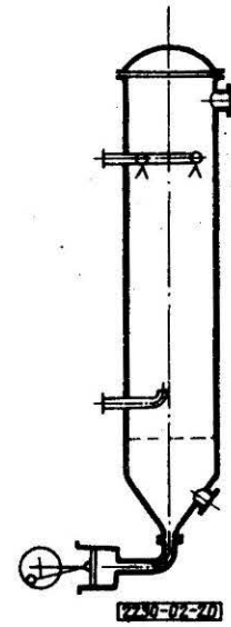
Rys. 20. Kolumna pulsacyjna
