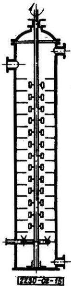
Rys. 15. Kolumna wirnikowa z wirującymi mieszadłami
