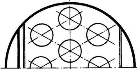
Rys. 4. Półki z kołpakami dzwonkowymi
