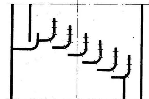
Rys. 11. Półki szczelinowe 2230-02-11
