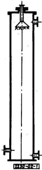
Rys. 1. Kolumna bez wypełnienia
