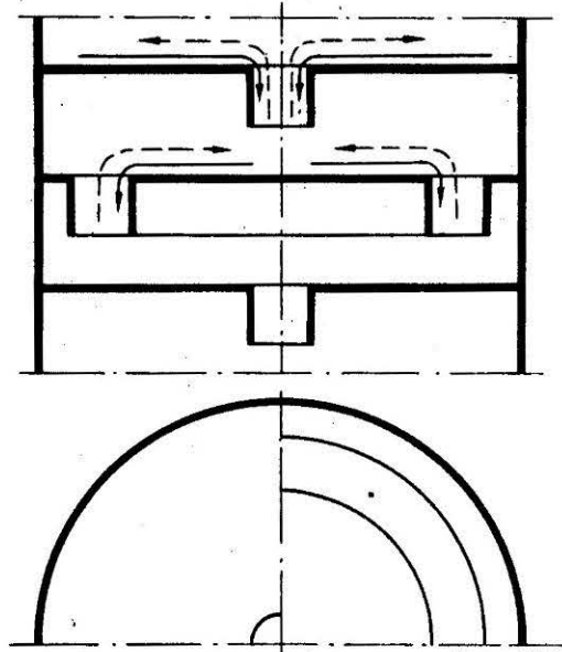
Rys. 14. Półka warstewkowa
