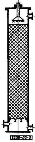
Rys. 2. Kolumna z wypełnieniem
