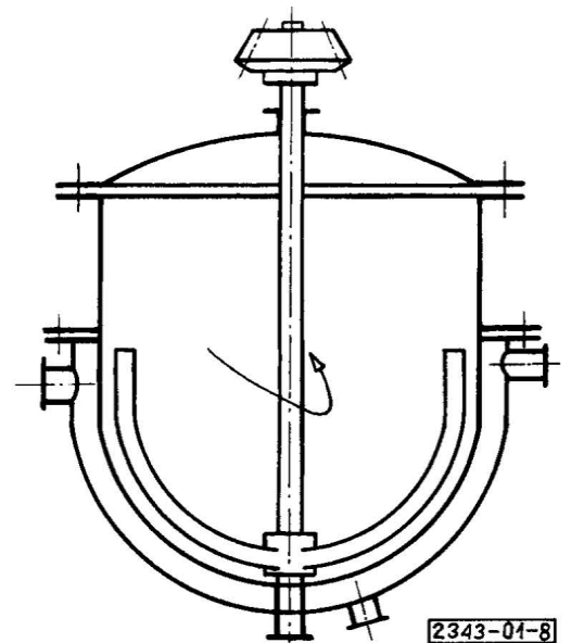
Rys. 8. Mieszarka pionowa z mieszadłami kotwicowymi
