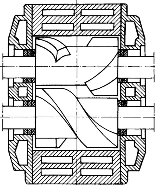
Rys. 2. Mieszarka zamknięta z mieszadłami śrubowymi
