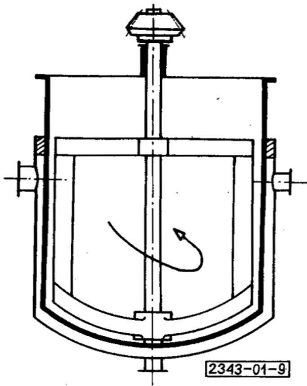
Rys. 9. Mieszarka pionowa z mieszadłami ramowymi
