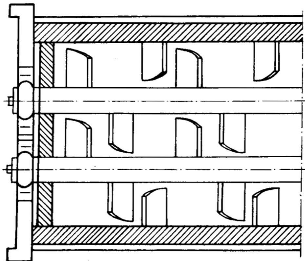
Rys. 5. Mieszarka pozioma z mieszadłami grzeblowymi
