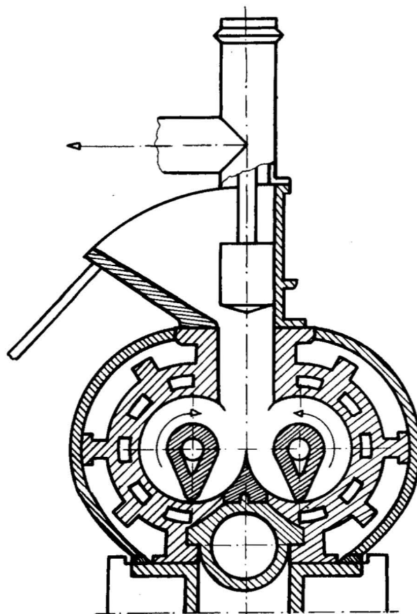
Rys. 1. Mieszarka zamknięta z mieszadłami owalnymi
