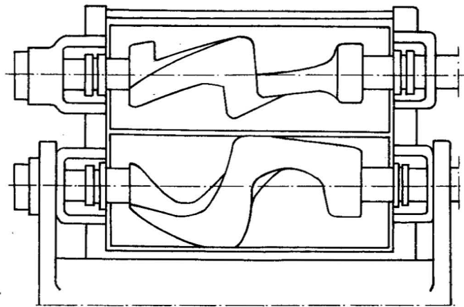
Rys. 4. Mieszarka pozioma z mieszadłami zetowymi
