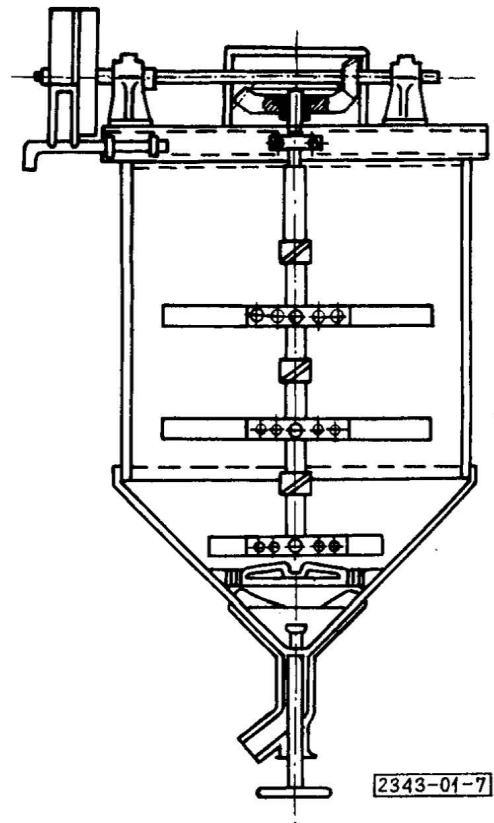
Rys. 7. Mieszarka pionowa z mieszadłami łopatkowymi
