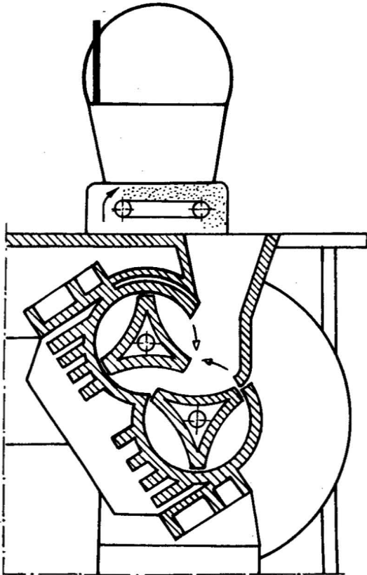
Rys. 3. Mieszarka zamknięta z mieszadłami trójgraniastymi
