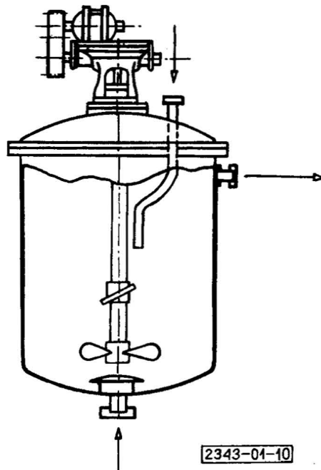
Rys. 10. Mieszarka pionowa z mieszadłami śmigłowymi
