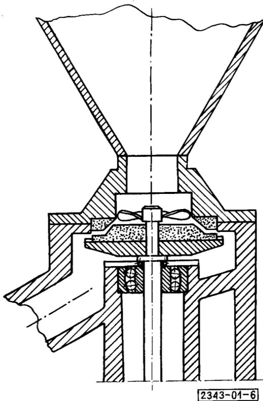
Rys. 6. Mieszarka pionowa z mieszadłami tarczowymi
