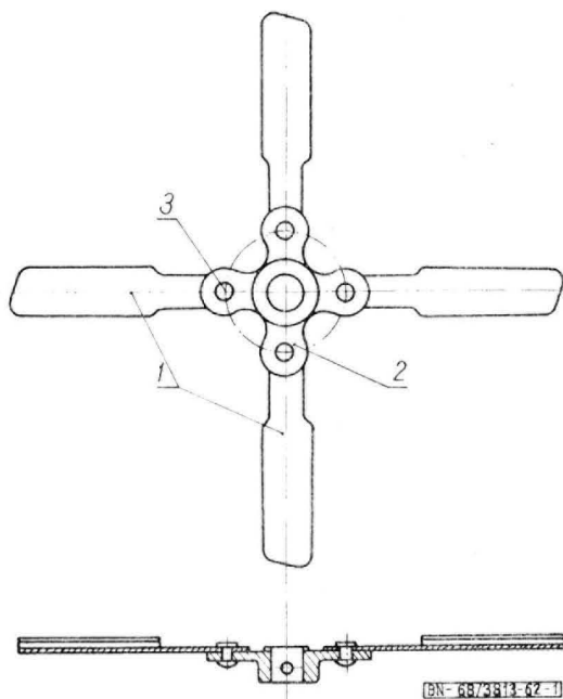
Rys. 1. Zamek krzyżowy
