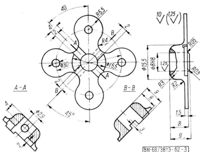
Rys. 3 Krzyżak
