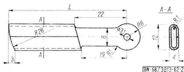
Rys. 2. Ramię
