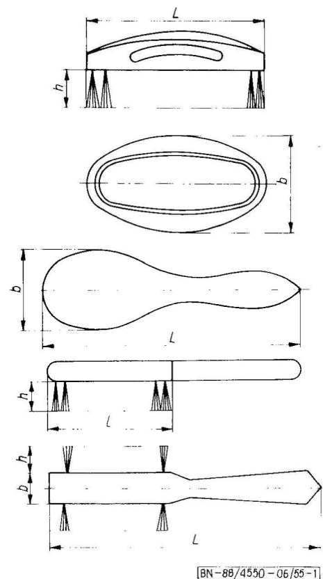
Rys. 1. Szczotki do włosów dla dorosłych
