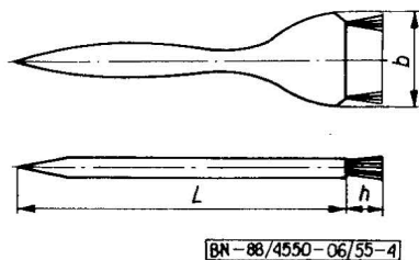
Rys. 4. Szczotka do farbowania włosów
