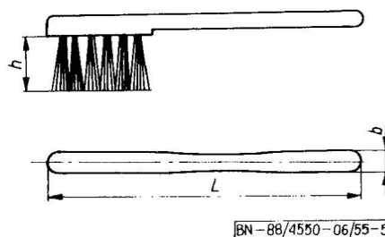
Rys. 5. Szczotka do rzęs
