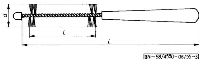
Rys. 3. Szczotka do włosów skręcana w drucie
