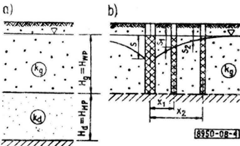
Rys. 4. Obliczanie k_g gdy u \geq 6 : a) układ warstw w przekroju, b) zastępczy schemat obliczeniowy
