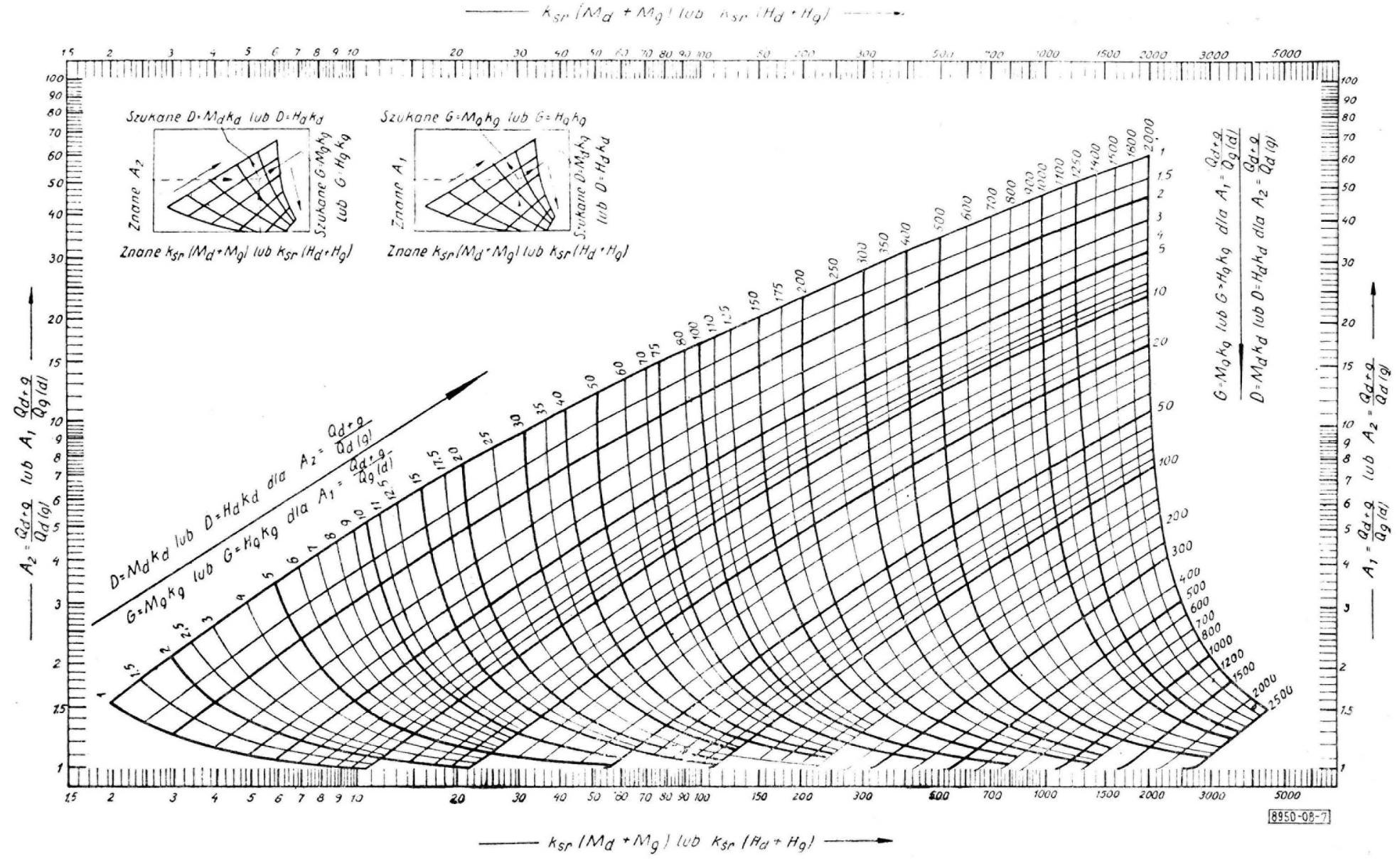
Rys. 7. Nomogram do wyznaczania wartości przewodności D=M_d k_d i G=M_g k_g lub D=H_d k_d i G=H_g k_g
