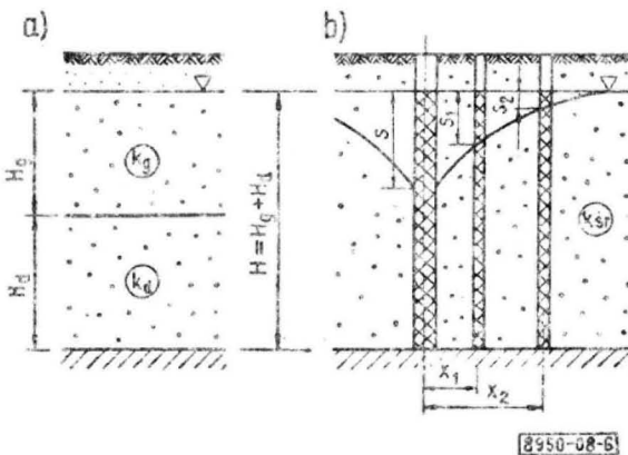
Rys. 6. Obliczanie k_{sr} : a) układ warstw w przekroju, b) zastępczy schemat obliczeniowy
