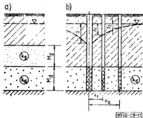
Rys. 11. Obliczenie k_d gdy k'_d > 10 k'_g : a) układ warstw w przekroju, b) zastępczy schemat obliczeniowy
