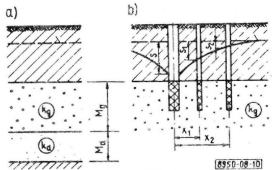
Rys. 10. Obliczanie k_d gdy k'_d > 10 k'_g : a) układ warstw w przekroju, b) zastępczy schemat obliczeniowy
