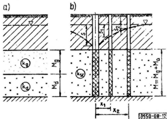
Rys. 12. Obliczenie k_{sr} : a) układ warstw w przekroju, b) zastępczy schemat obliczeniowy
